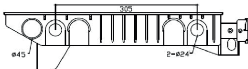
DPI-1452 3 X 18 1/2 F-SERIES 85-96
