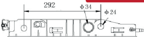
DPI-2353 2 3/8 X 18 5/8 CAMARO 3.3L V6 93
