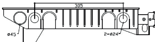
DPI-1452 3 X 18 1/2 F-SERIES 85-96
