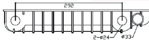
DPI-888 2 3/8 X 16 7/16 AUT./T BLAZER/S-10 83/90
